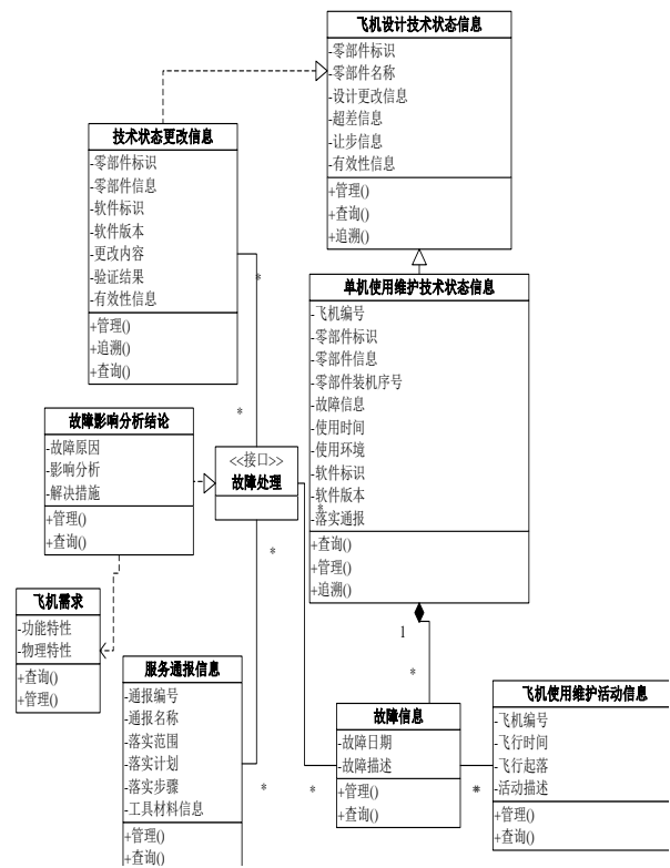
图 3 军用飞机复杂故障处理 UoF(功能单元)模型
