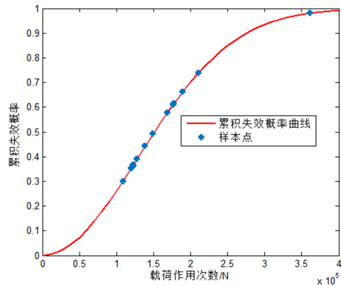
图 3 整体搭接壁板结构疲劳寿命分布曲线
