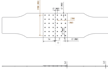
图 1 试验件几何结构形式图
